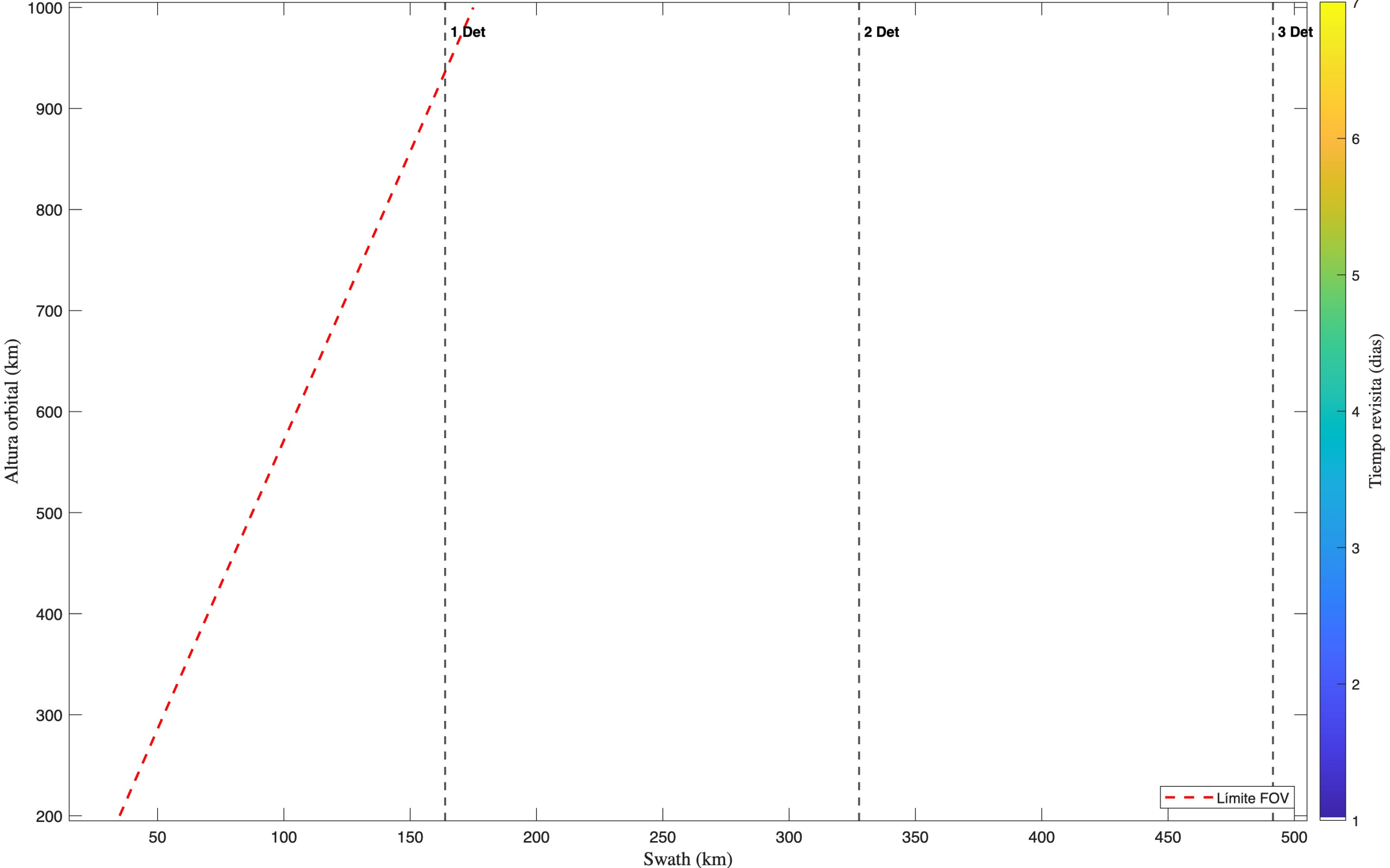
Tiempo Revisita - 1 Satelite(s); 1 Telescopio(s): Refractivo; Detector 2 (Blanco: \geq 7 dias)
